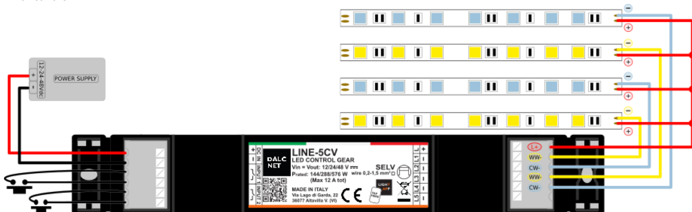
Figura 3: Schema di collegamento per carichi LED Bianco-Dinamico
