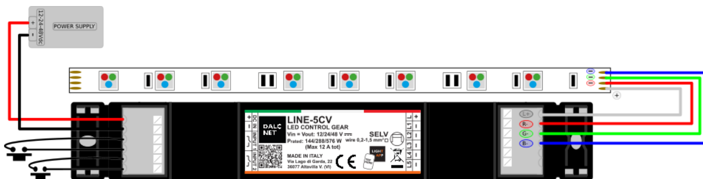
Figura 4: Schema di collegamento per carico RGB
