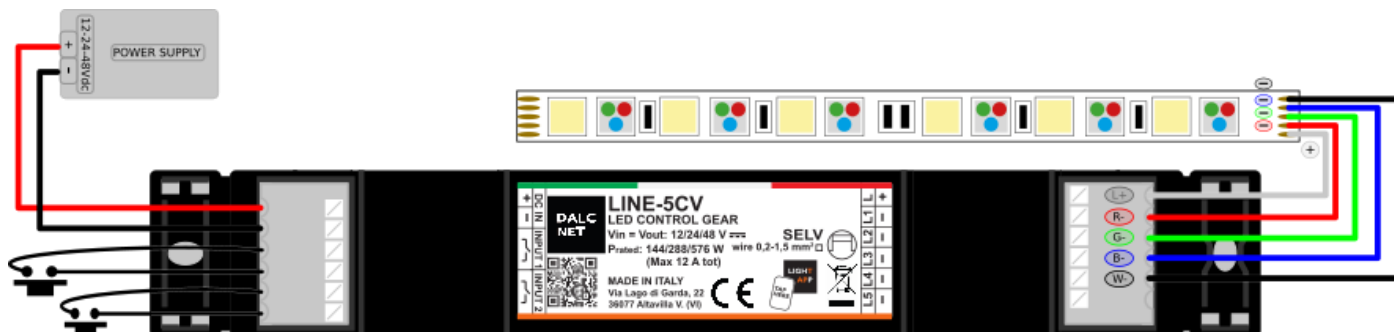
Figura 5: Schema di collegamento per carico LED RGBW
