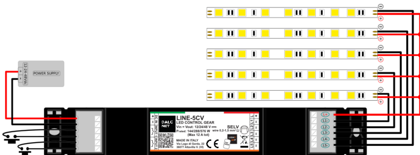
Figura 2: Schema di collegamento per carichi LED Bianchi o Monocolore
