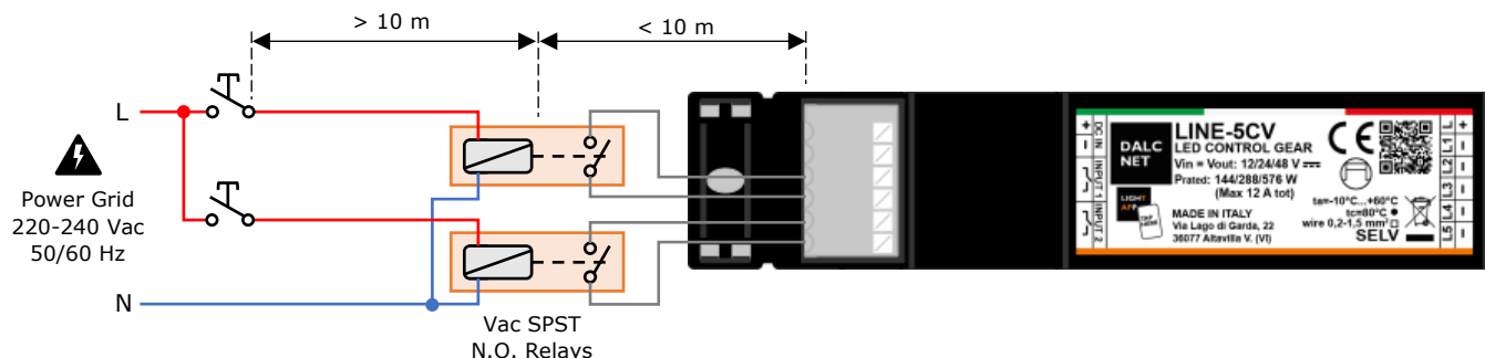
Figura 8: Collegamento del Comando Locale per lunghe distanze
