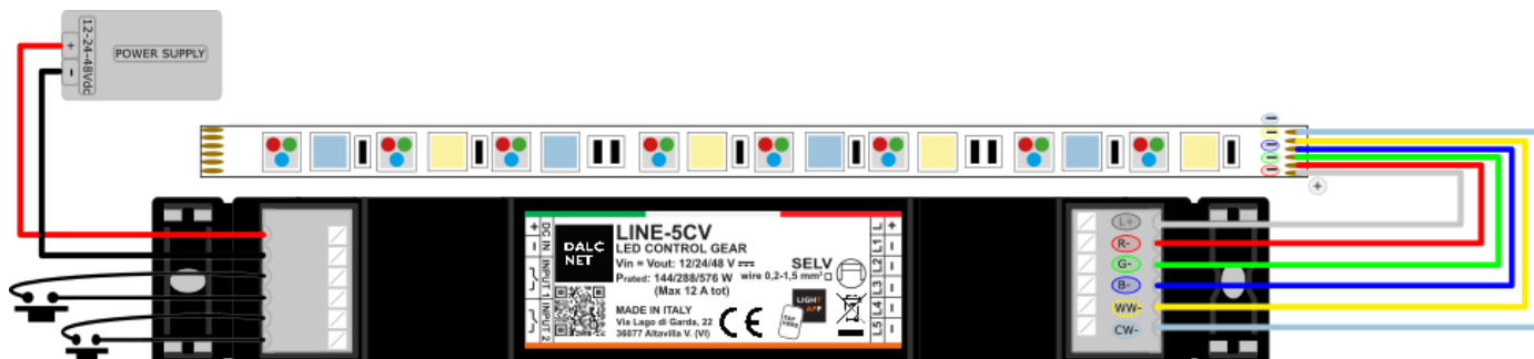
Figura 6: Schema di collegamento per carico LED RGB+TW
